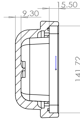
A-A 比例 1 : 3
